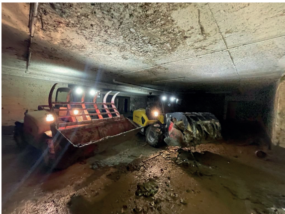
Odstranjanje blata in odpadkov z dvema našima teleskopskima vozičkoma
